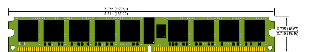
VLP RDIMM MO-237 240 PIN
