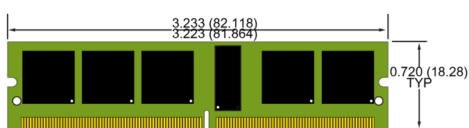
MINI R-DIMM VLP MO-244 244 PIN
