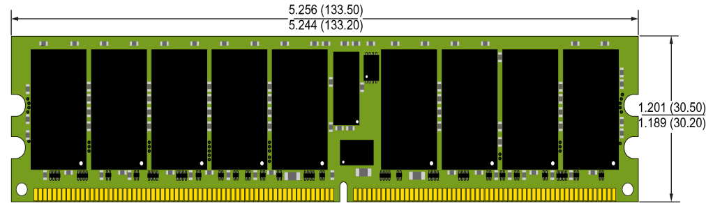
RDIMM MO-237 240 PIN
