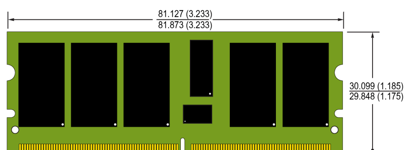
MINI R-DIMM MO-244 244 PIN
